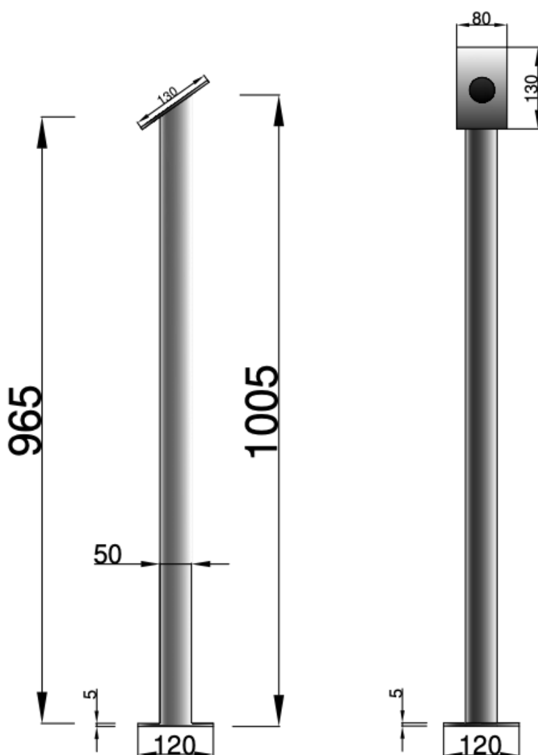
SŁUPEK POD CZYTNIK 130X85 STAL 304 N SZLIF nr katalogowy 10007
